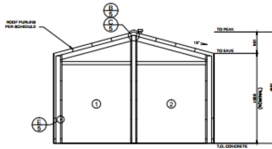
4 ENDWALL INTERIOR ELEVATION SCALE: 1:100
