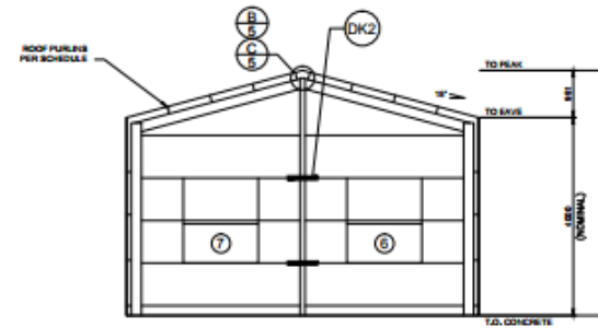
3 ENDWALL INTERIOR ELEVATION SCALE: 1:100
