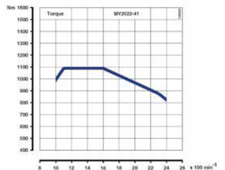
PACCAR PX-7 212
