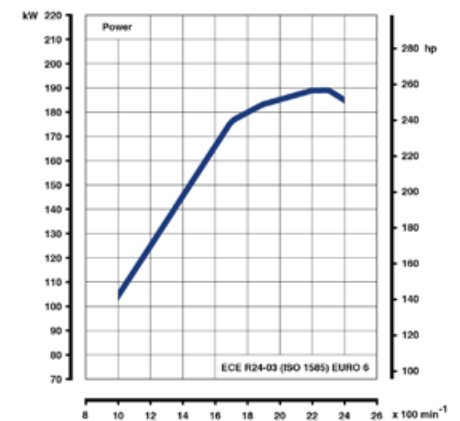
PACCAR PX-7 212
