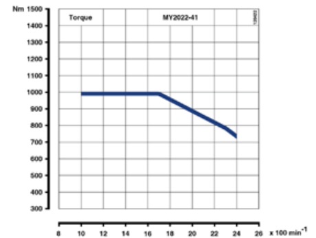
PACCAR PX-7 189
